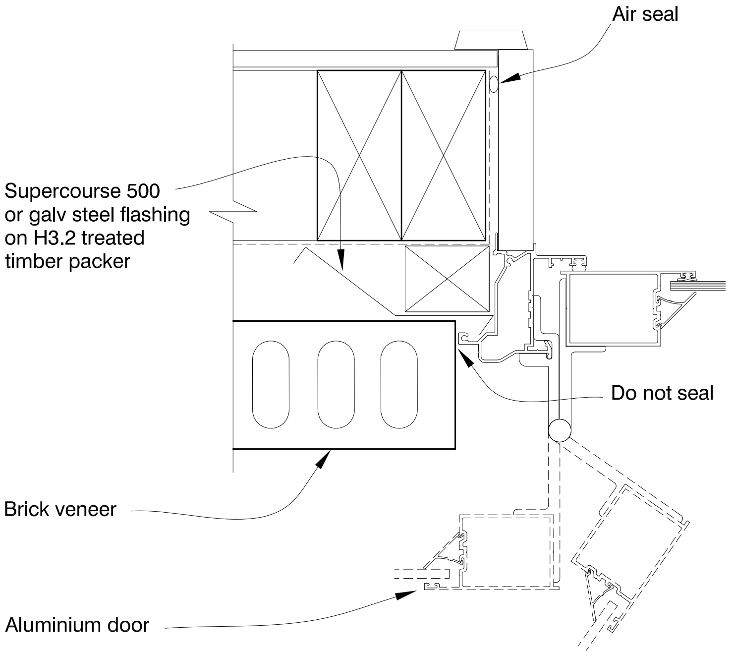
FIG. 39 DOOR JAMB - Aluminium
