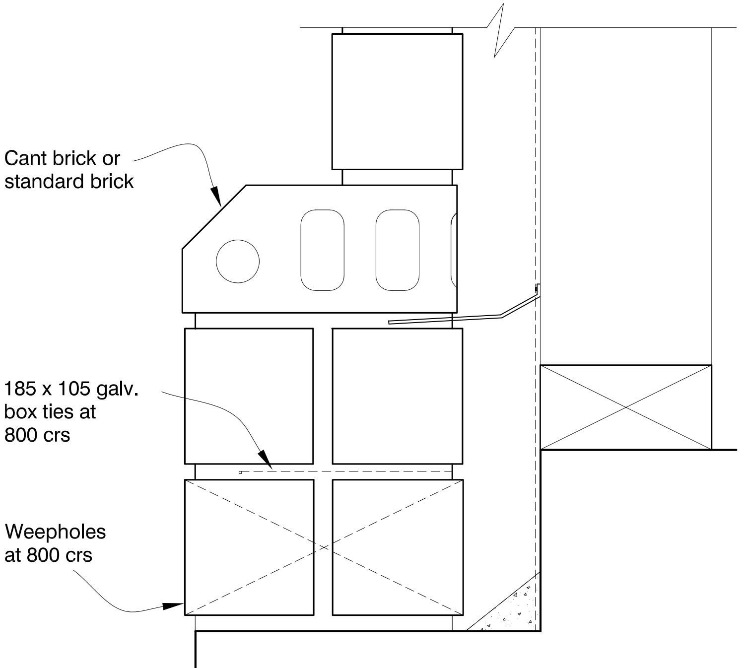
FIG. 11 PLINTH BASE
