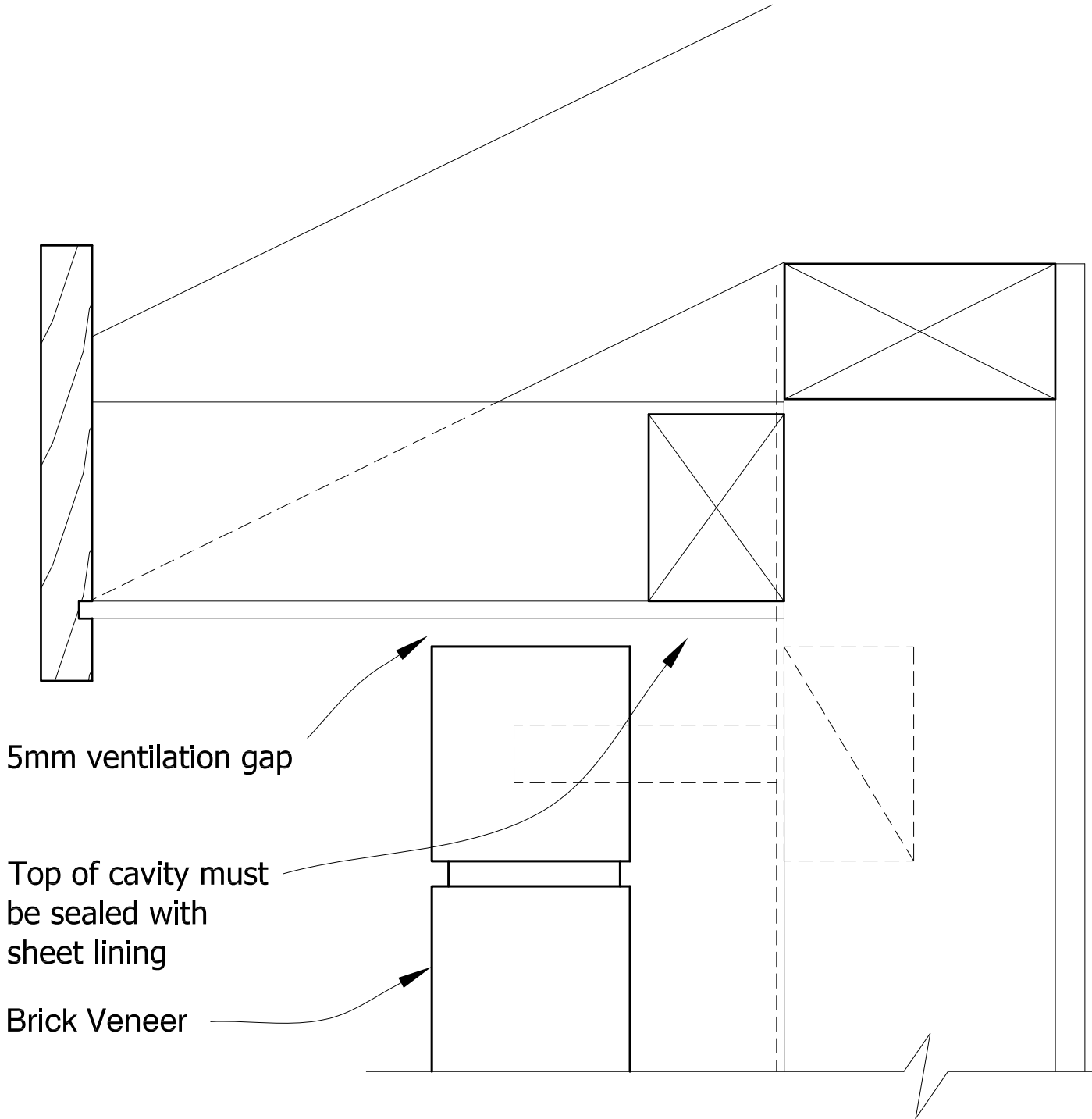
FIG. 4 FLAT SOFFIT
