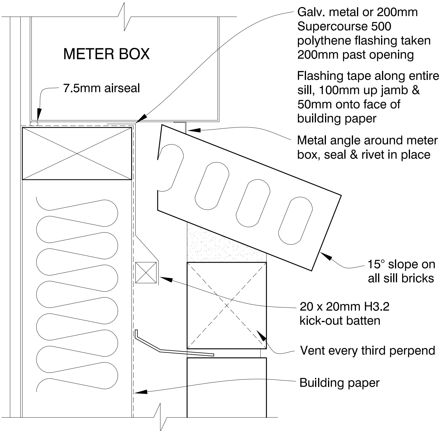
FIG. 73 METER BOX SILL
